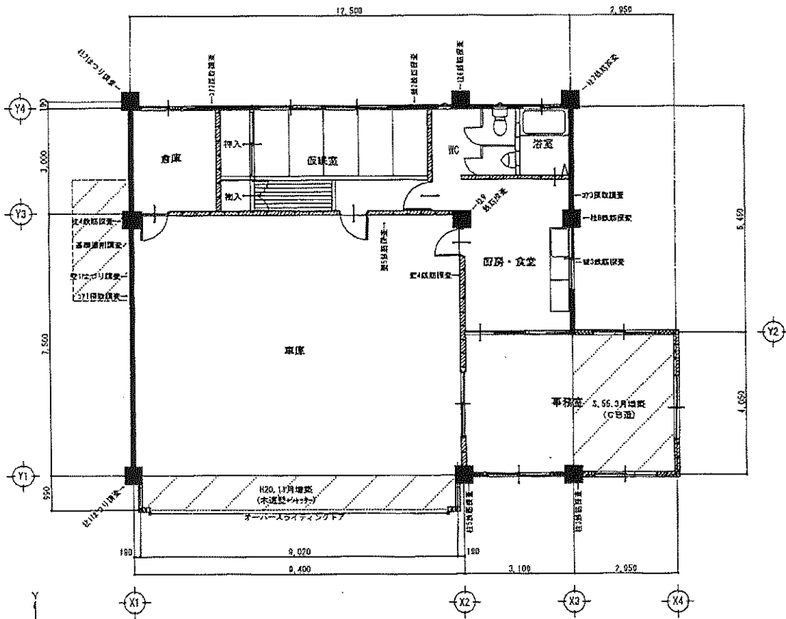
平面図 S-1/100
